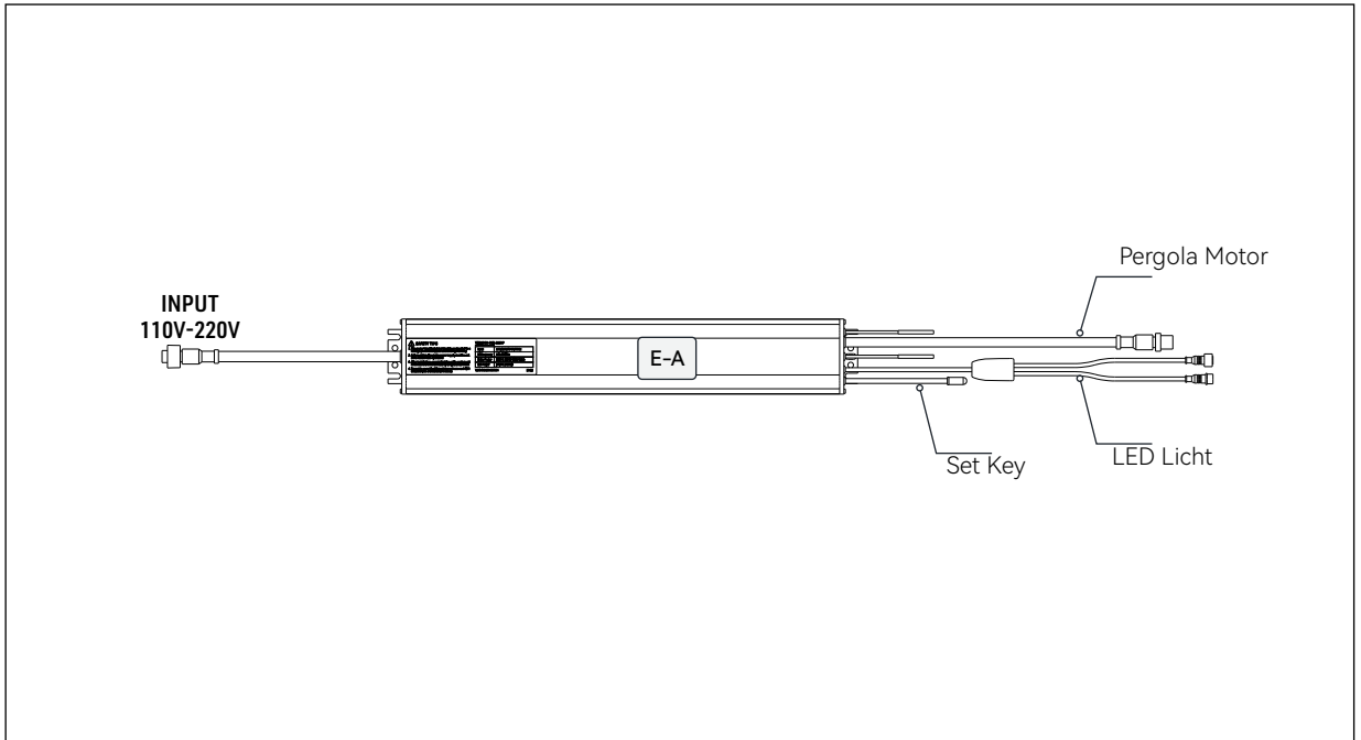
Kabelbild
