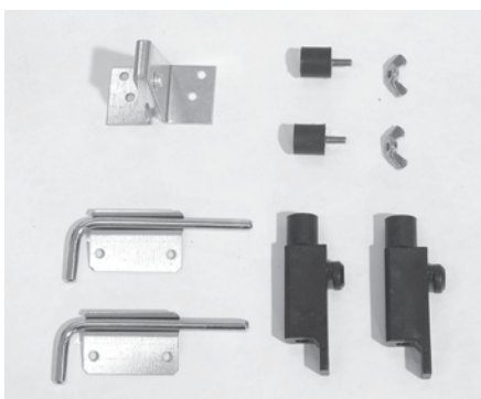
Stopper, Gummipuffer, Verriegelung, Umlenkrolle, Flügelmutter Stopper, rubber buffer, locking, guide pulley, wingnut Arrêt-ressort, arrêts en caoutchouc, serrure verrouillage, poulie, écrou à oreilles Katrol, rubber stoppers, veer stoppers, ...
